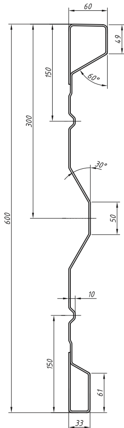
Zeichnung SU-600/60/33
