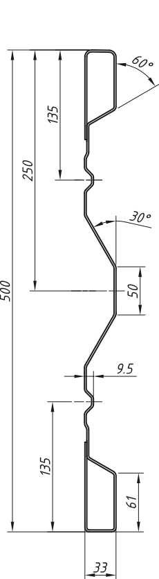
Zeichnung SU-500/33/33
